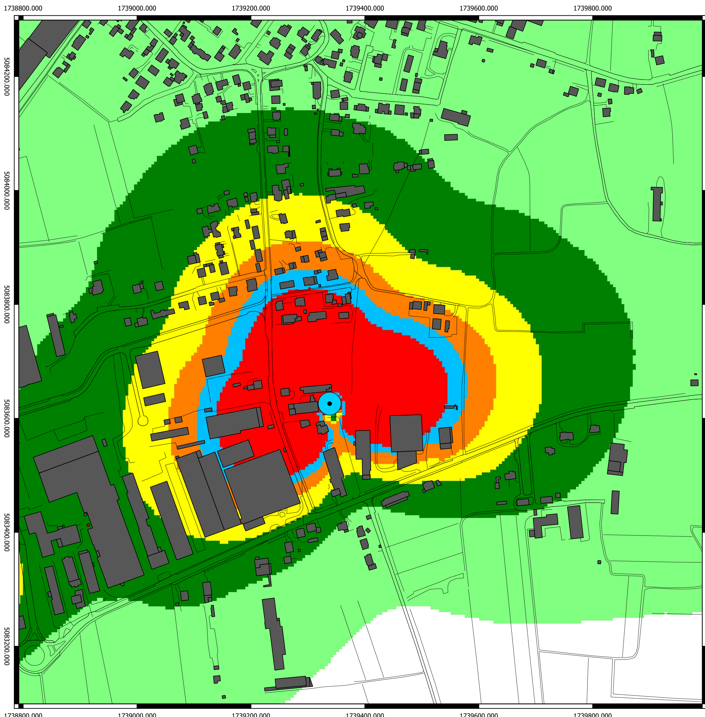
Campo elettromagnetico (V/m) calcolato alla quota di 15,5 m sul livello del terreno
