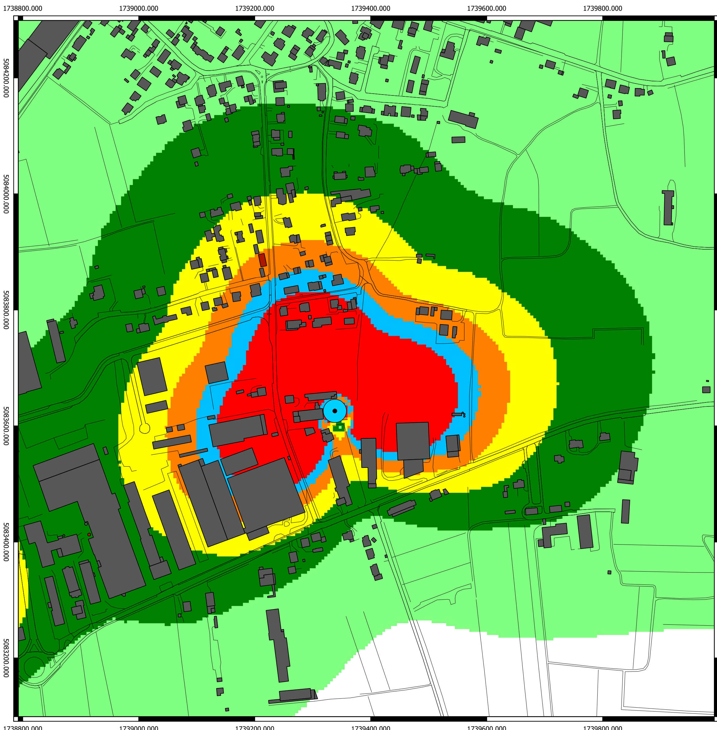
Campo elettromagnetico (V/m) calcolato alla quota di 13,5 m sul livello del terreno
