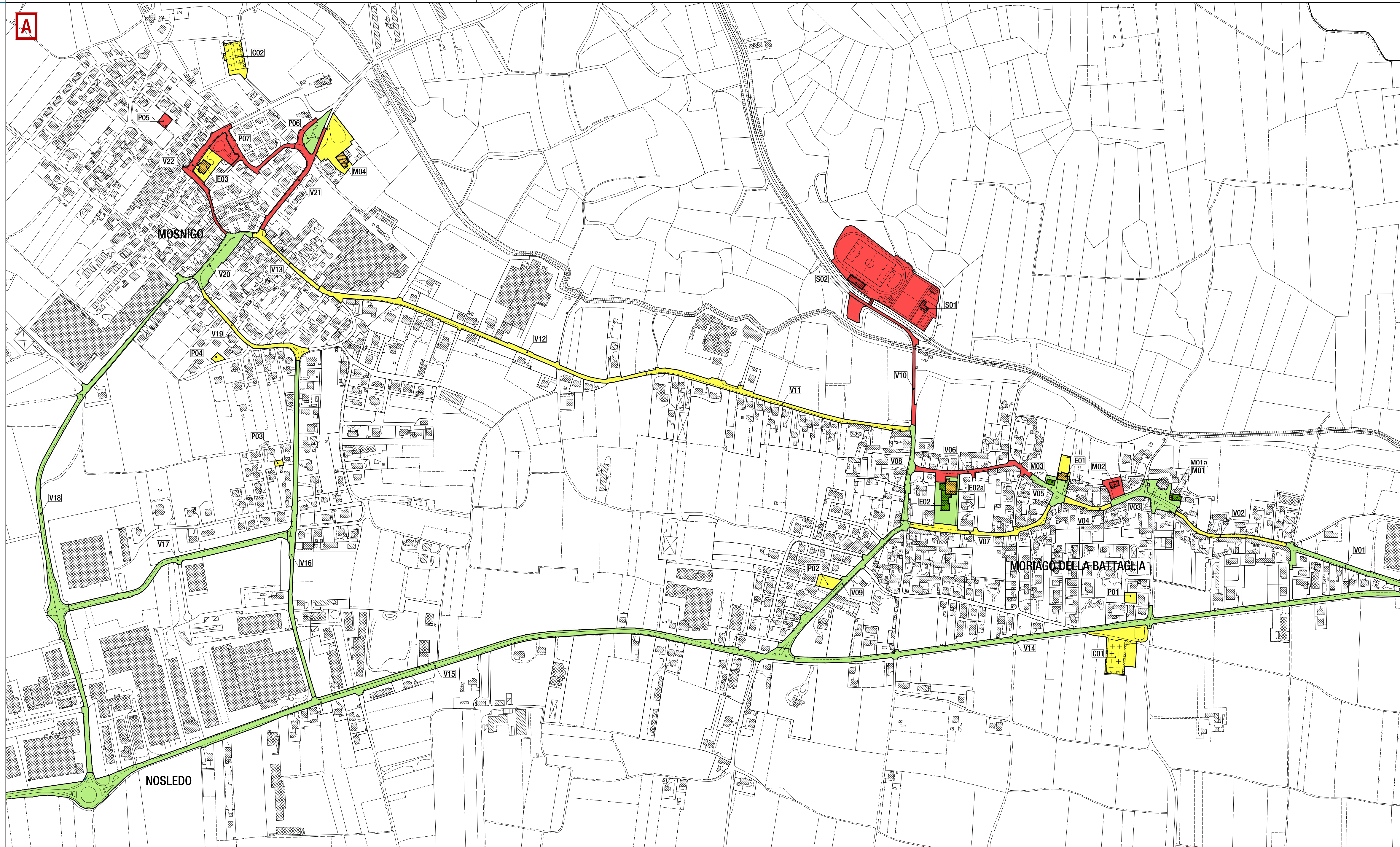
PLANIMETRIA STATO DI FATTO - GRADO DI ACCESSIBILITÀ - AREA A
